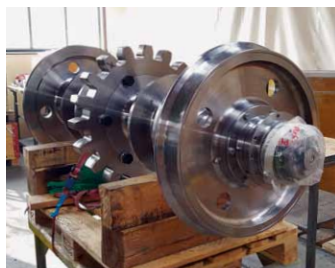
Bremsradsatz
